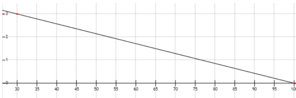
Función z (b)
